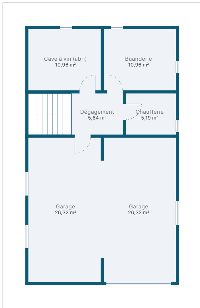
Sous-sol garages – buanderie – technique
